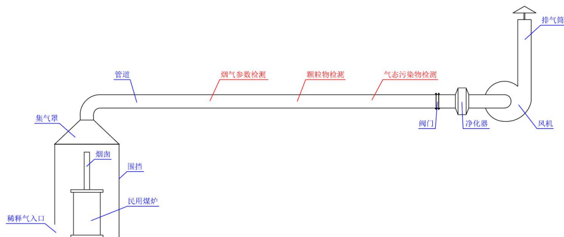
图 B.1 民用煤大气污染物排放系数检测平台示意图
